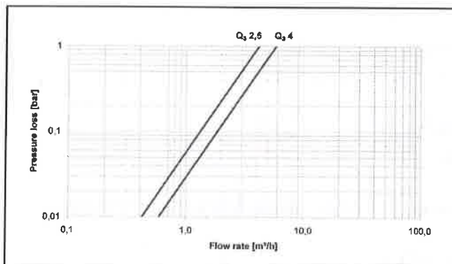
Nyomásveszteség diagram
